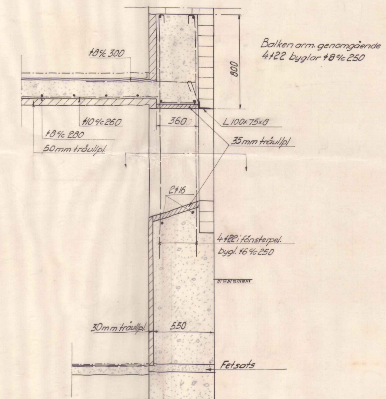
Sektion P-P
