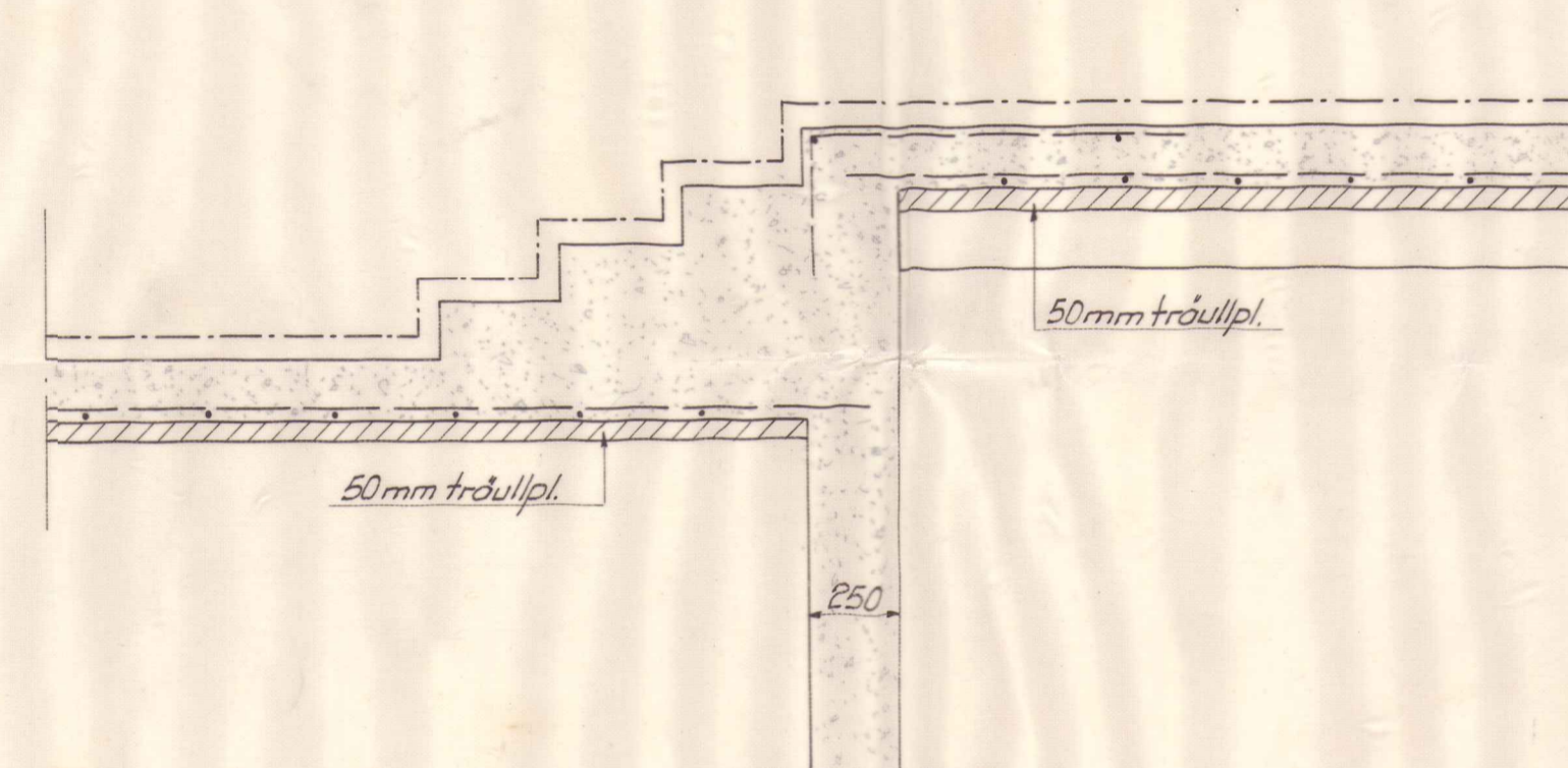
Sektion O-O
