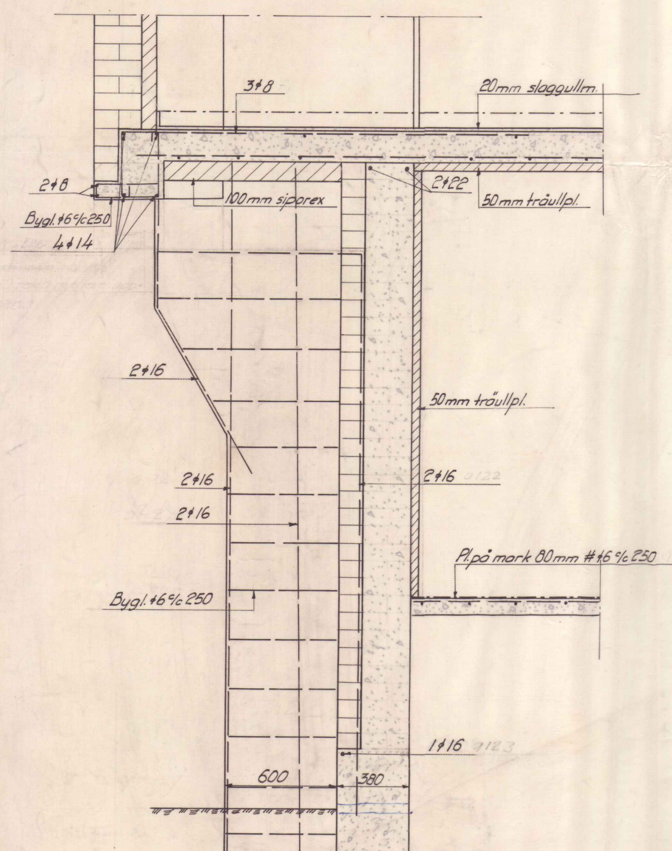
Sektion F-F
