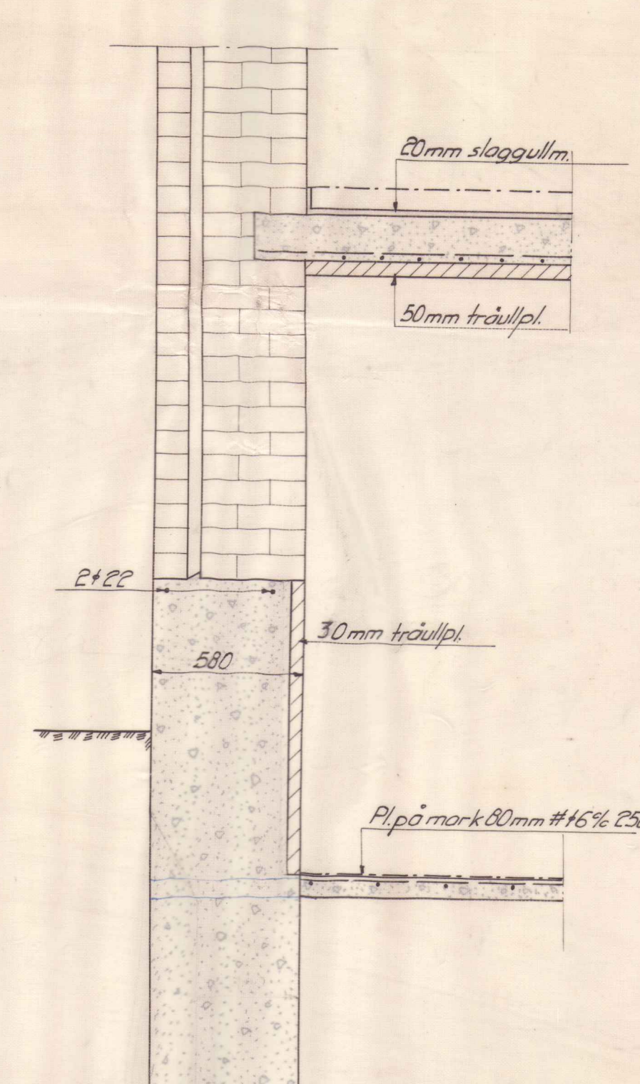
Sektion I-I
