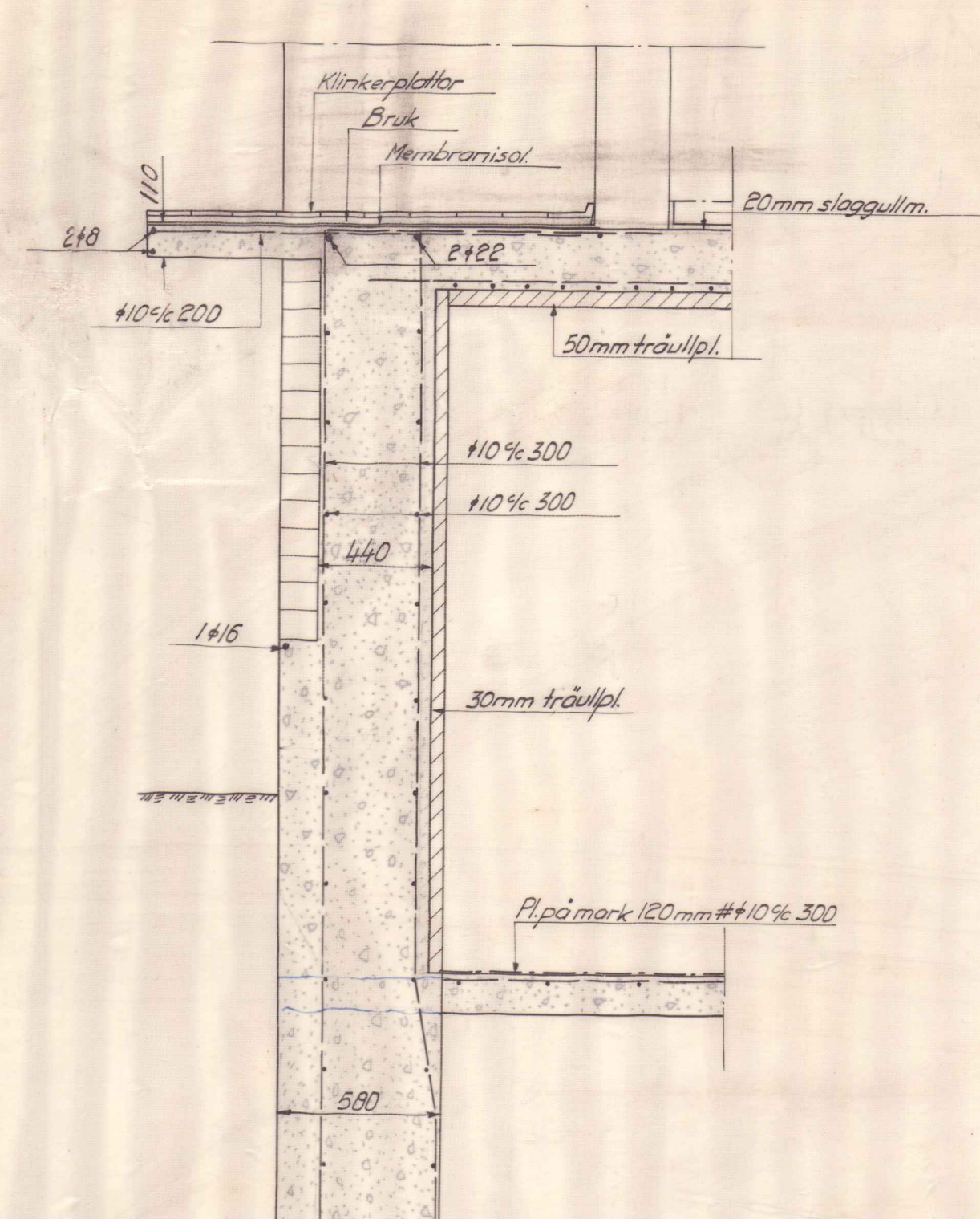
Sektion H-H
