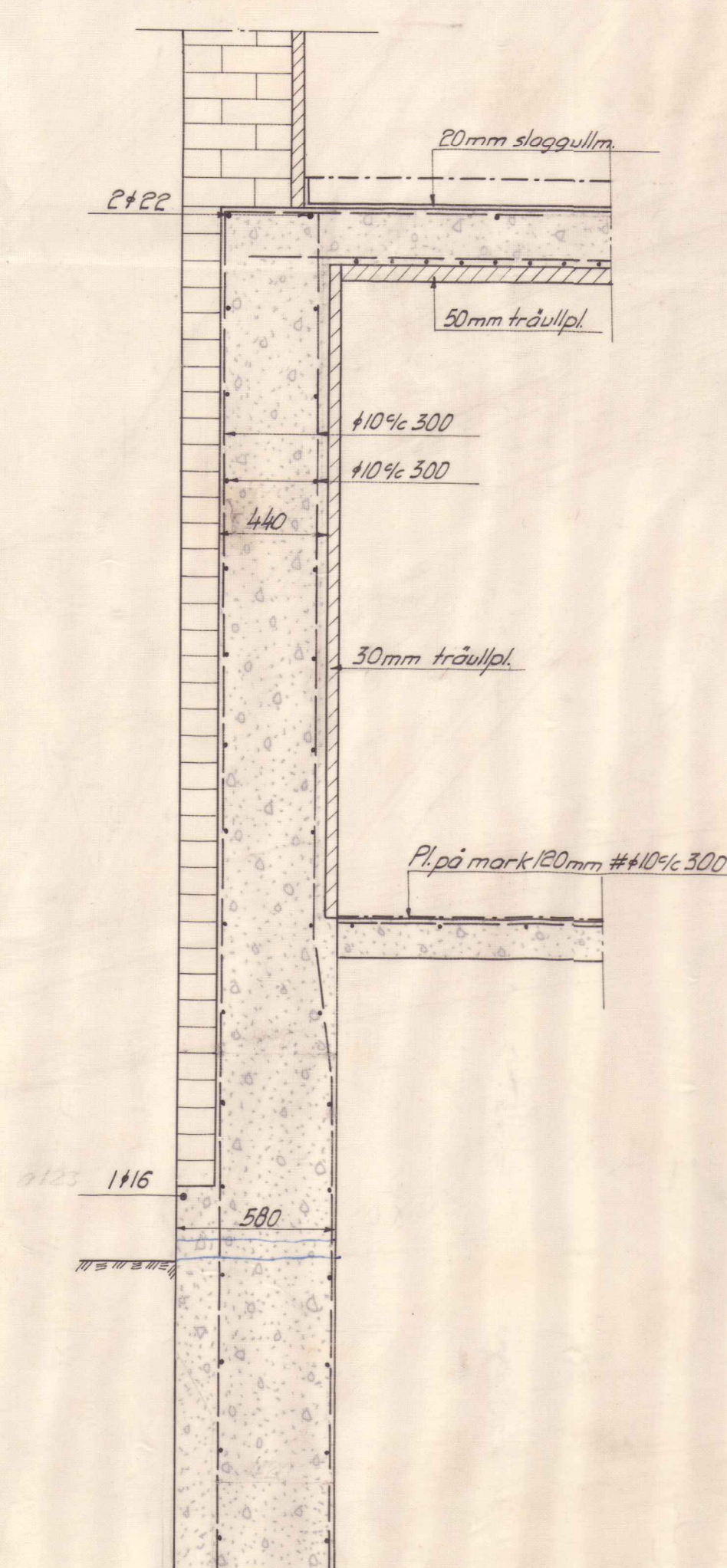
Sektion G-G
