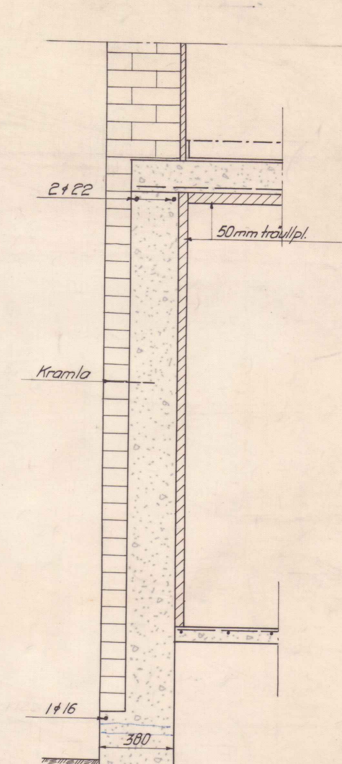
Sektion J-J
